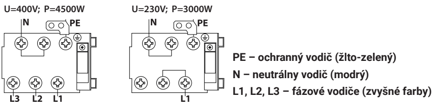
Obr. 2 – Schéma zapojenia
