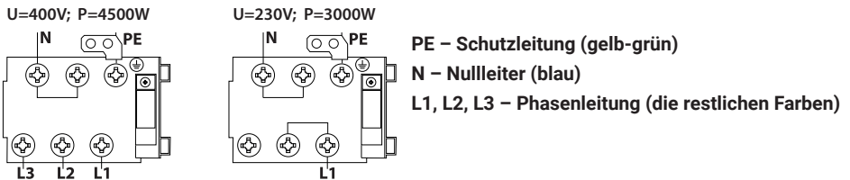
Abb. 2 - Etikette mit dem Schaltplan
