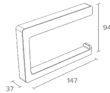
793003 - schwarz / black matt 794003 - weiß / white matt Papierrollenhalter / Toilet Roll Holder
