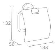
740006 Papierrollenhalter / Toilet Roll Holder
