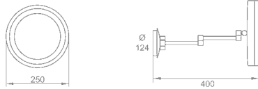
020801 LED CITY LIGHT SMD-LED-Beleuchtung 3-fach-Vergrößerung Doppel-Schwenkarm / SMD-LED-lighting 3x magnification Twin Arm
