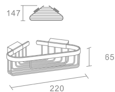
030706 Eckseifenkörbchen Messing mit Pulverbeschichtung / Corner Soap basket Brass with powder coating
