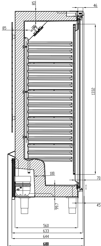
Masszeichnung Backwarenkühlschrank BKU 460 [Art. 45110460]
