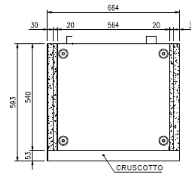
SEZIONE D-D
